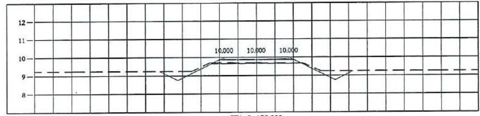
STA. 0+150.000 NGL = 9.700
