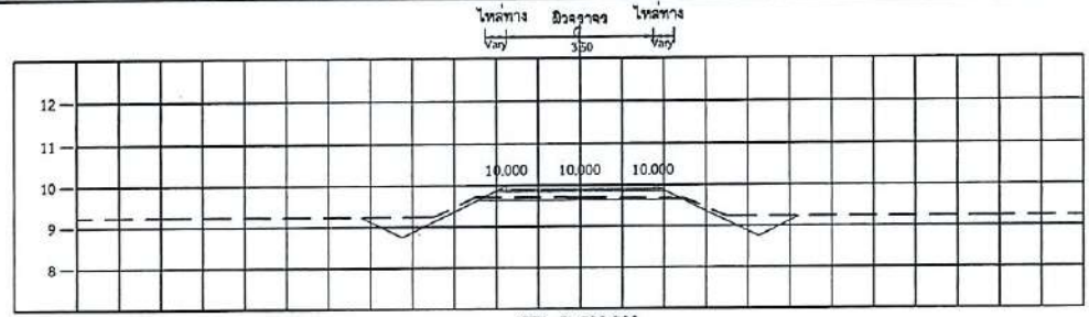
STA. 0+200.000 NGL = 9.710
