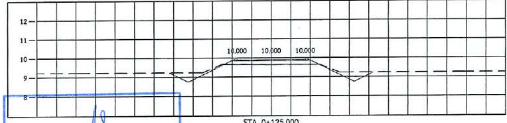
STA. 0+125.000 NGL = 9.641
