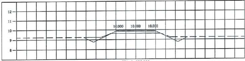
STA. 0+075.000 NGL = 9.635
