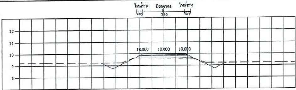
STA. 0+100.000 NGL = 9.620
