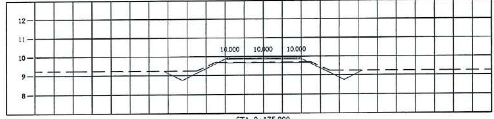
STA. 0+175.000 NGL = 9.680
