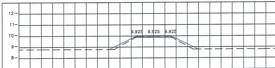
STA. 0+000.000 NGL = 9.825
