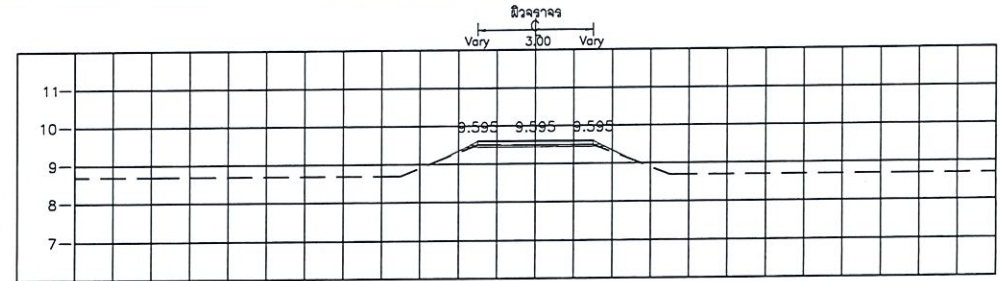
STA. 0+200.000 NGL = 9.495
