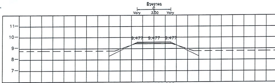
STA. 0+100.000 NGL = 9.365
