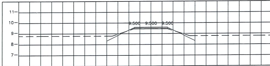
STA. 0+050.000 NGL = 9.350
